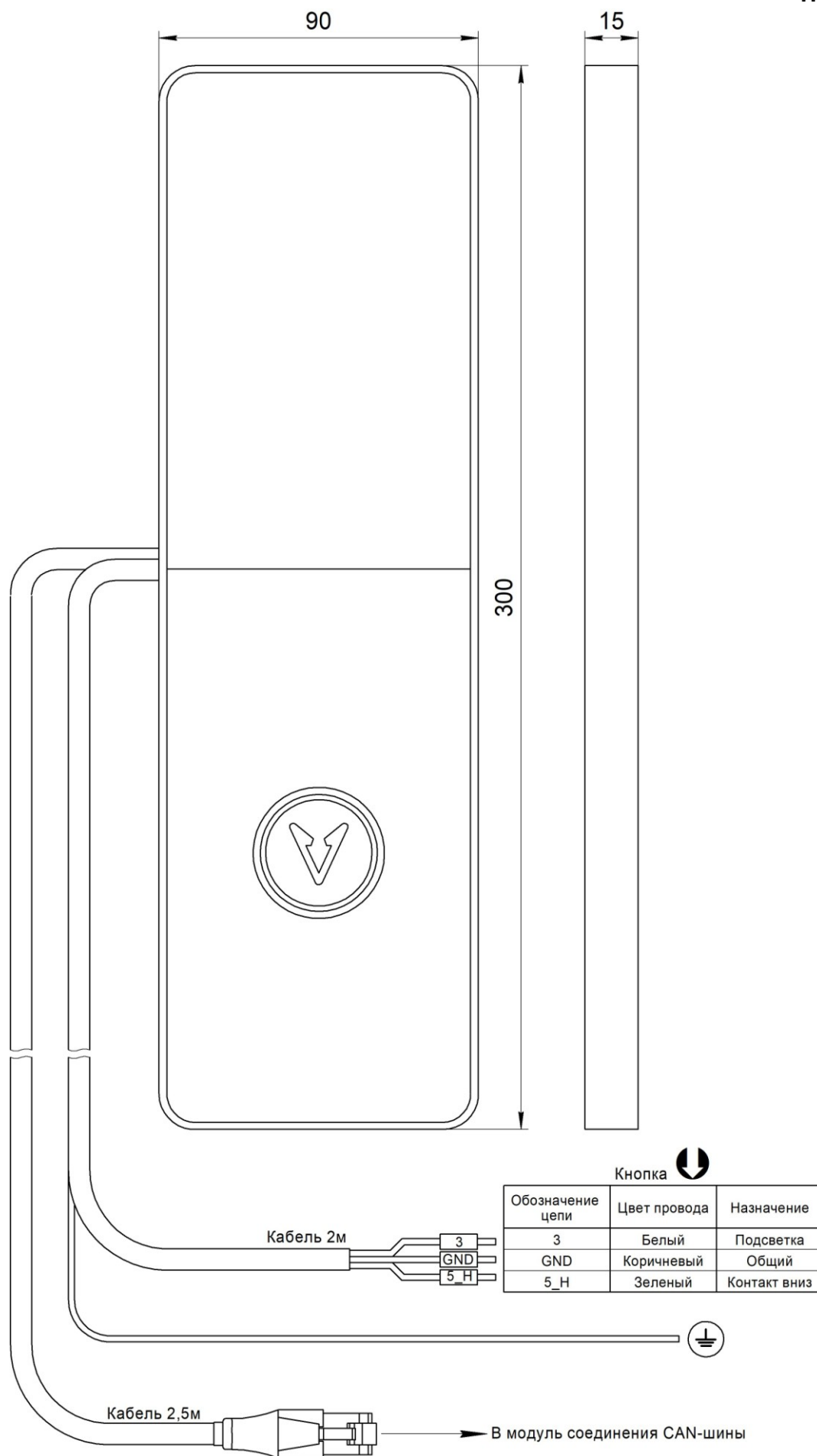
Рис.1 Внешний вид Вызывной пост ОПАЛ (жгут RJ45) НШЕК.468381.056-01
